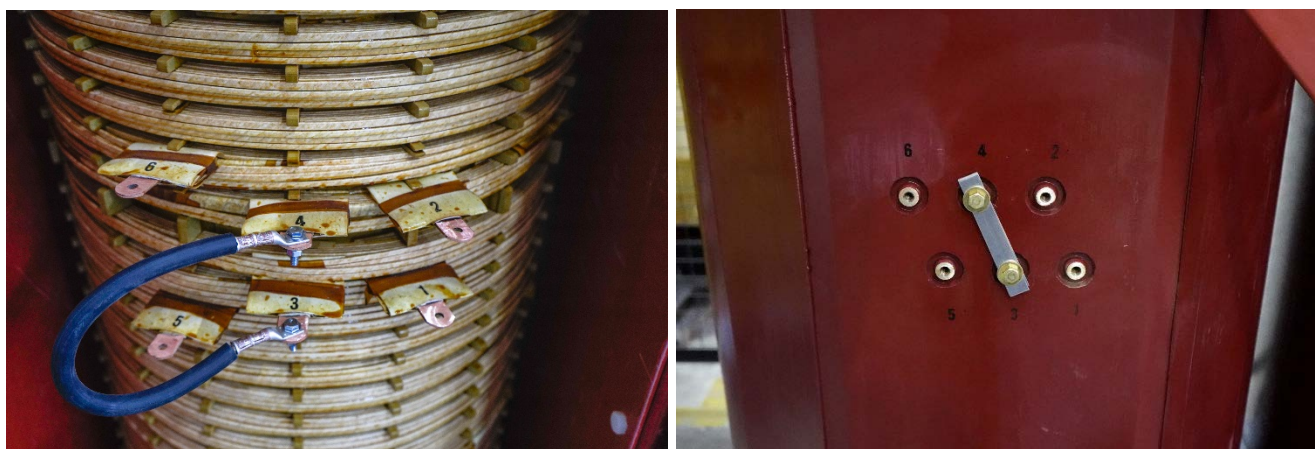
Figure 8: Gauche: prises de tension typiques sur la face de bobine pour le transformateur VPI. Droite : prises de tension typiques sur la face de bobine pour le transformateur de bobine coulé
