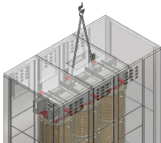
Figure 4: Chaînes de levage reliées au support de levage du transformateur.
